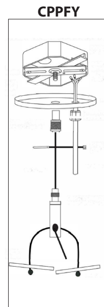
Cord Pendant Y-Hanger (Power Feed Capable)
